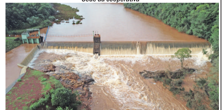
Usina CGH Buricá, localizada no Rio Buricá
