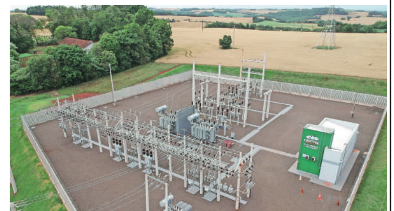
Subestação Nossa Senhora do Carmo foi inaugurada em 2021
