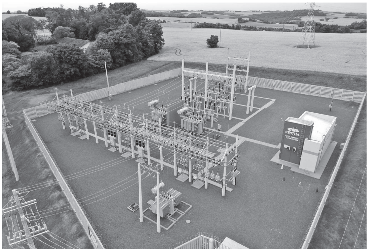
Inaugurada em 2021, a Subestação Nossa Senhora do Carmo - 69kV - considerada um marco na história da Certhil, proporciona uma maior disponibilidade de energia aos associados da cooperativa
